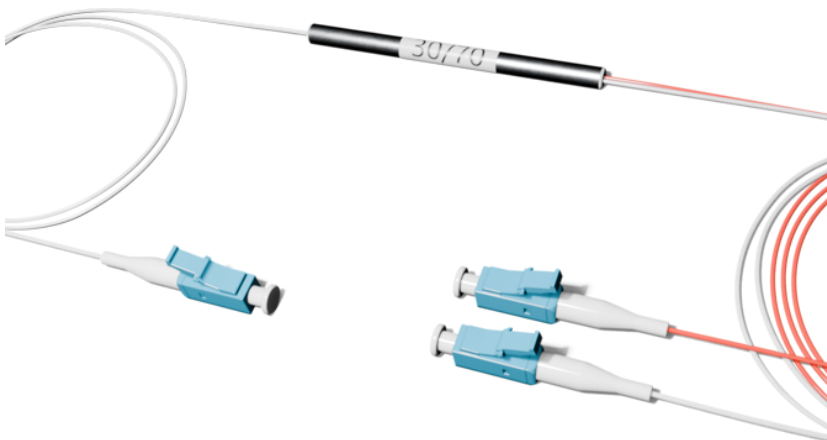
Рисунок 1 - Общий вид
