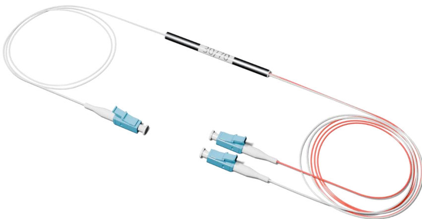
Рисунок 2 - Общий вид
