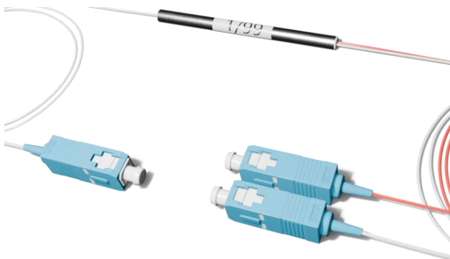
Рисунок 1 - Общий вид
