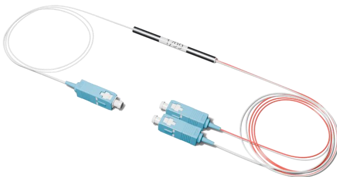
Рисунок 1 - Общий вид
