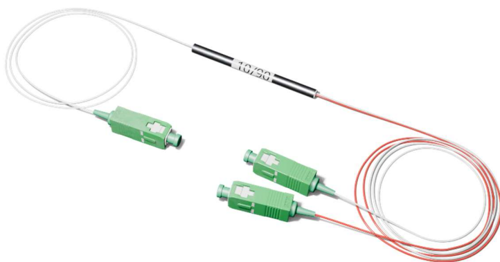
Рисунок 2 - Общий вид
