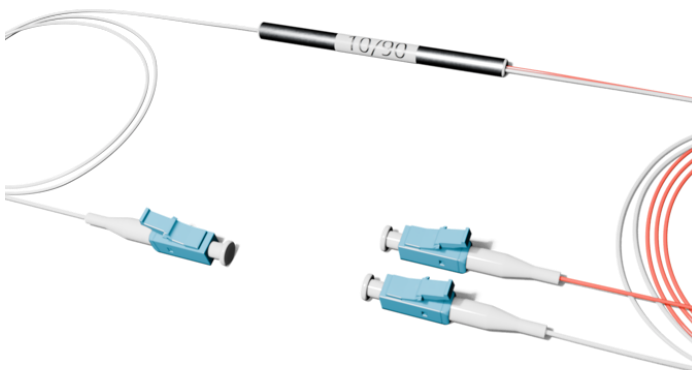
Рисунок 1 - Общий вид
