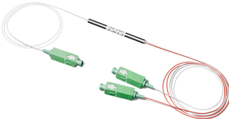
Рисунок 2 - Общий вид
