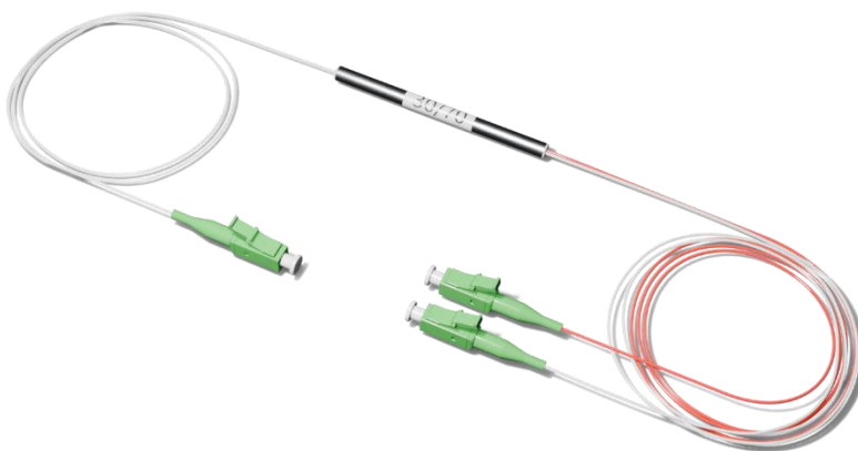
Рисунок 2 - Общий вид
